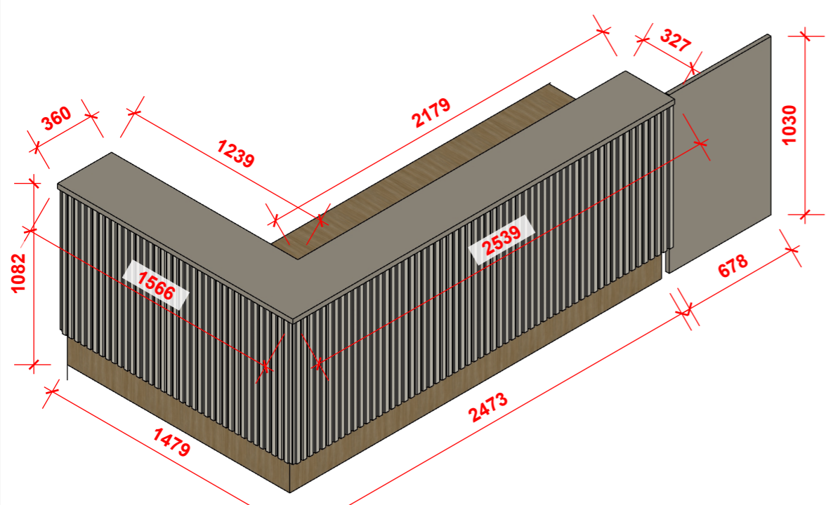
01 BALCÃO | PERSPECTIVA 1 ESC: 1/25
