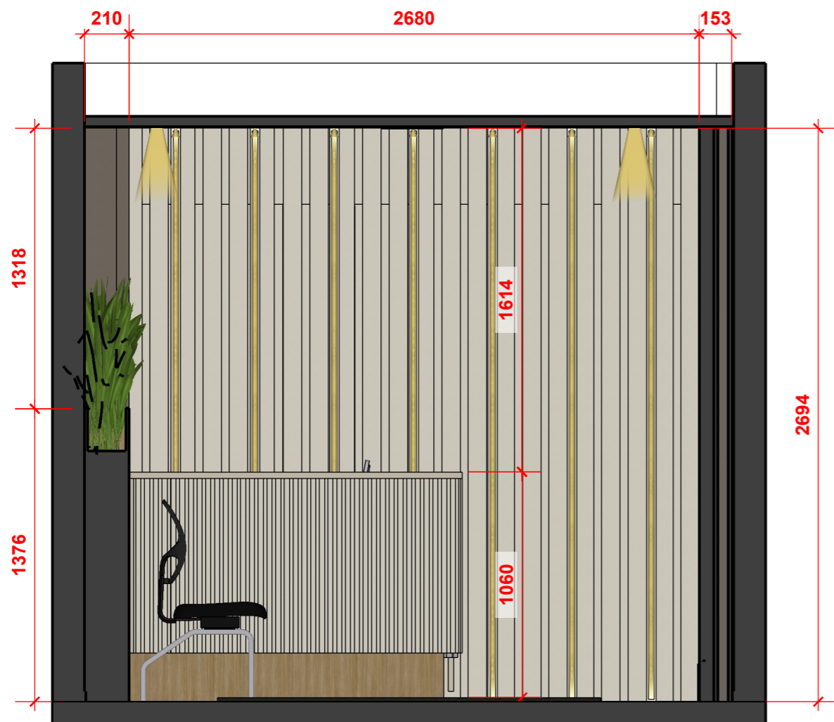
01 VISTA 03 ESC: 1/25
