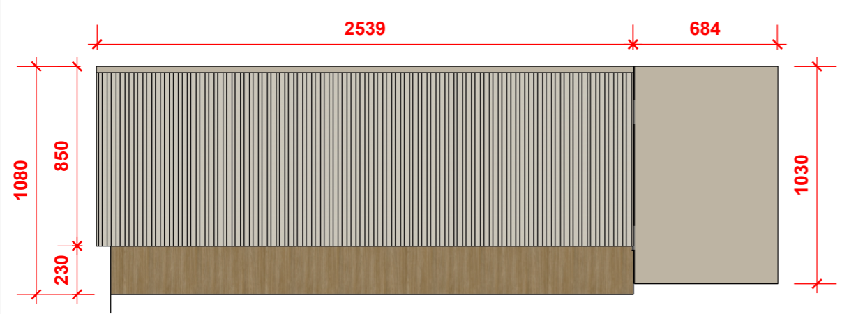
02 BALCÃO | FRONTAL ESC: 1/25
