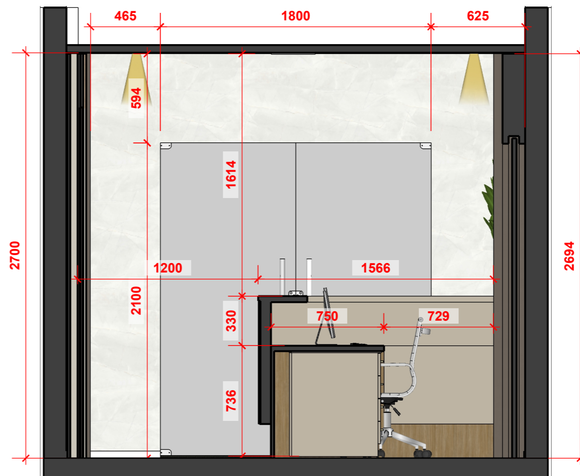
02 VISTA 04 ESC: 1/25
