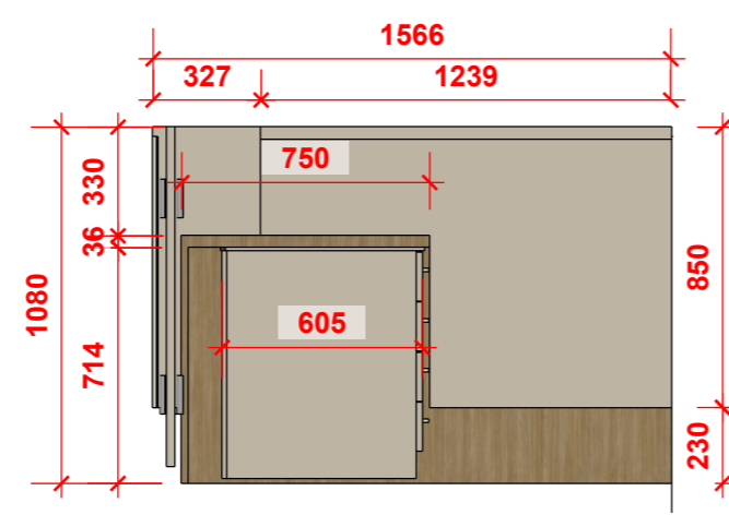
06 BALCÃO | LATERAL INTERNO ESC: 1/25
